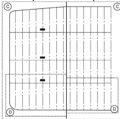
Petrolero: mamparo transversal típico
