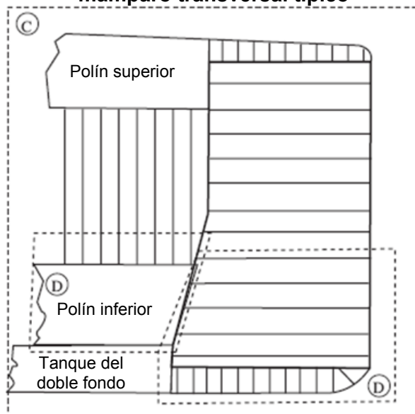
Mineralero/petrolero: mamparo transversal típico
