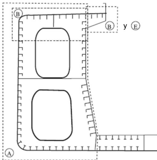
Mineralero/petrolero: sección transversal típica
