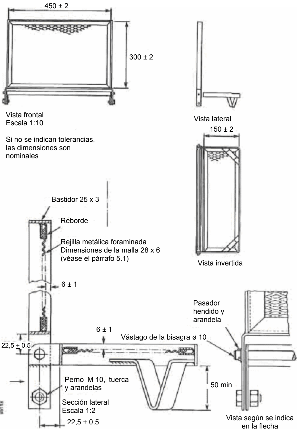
Figura 1 – Conjunto de prueba (Todas las dimensiones están expresadas en milímetros. Todas las piezas son de acero)
